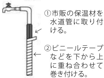
▲図1.水道管の防寒方法
