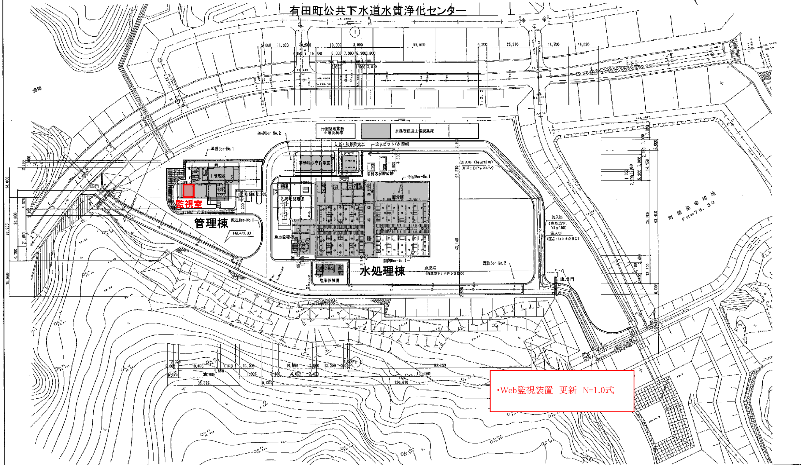
一般平面図 8-1:600
