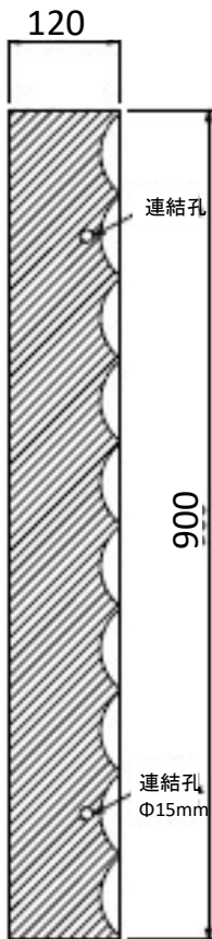
側面図
