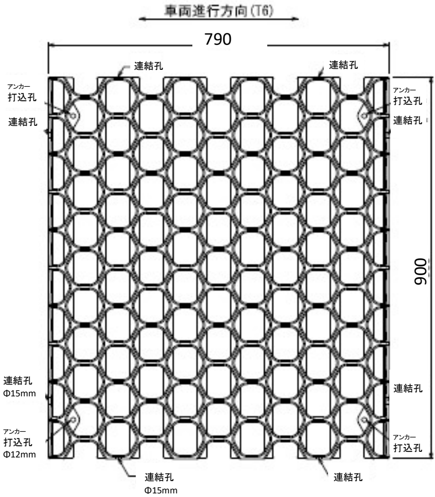
平面図
