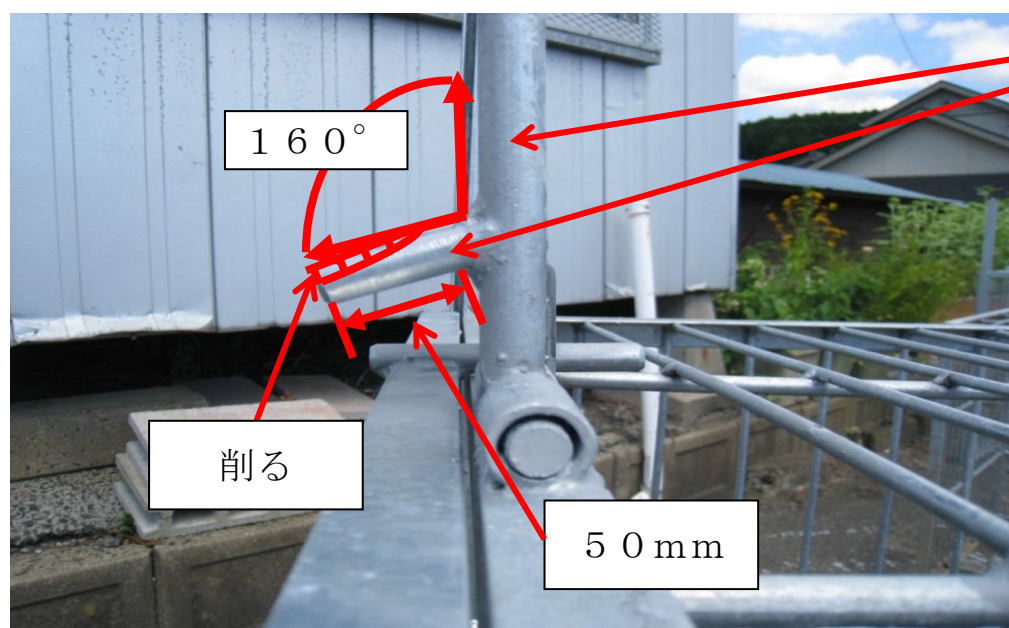
○側部からみた図面
