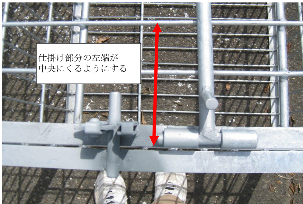
○上部からみた図面
