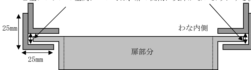
◎レール部分の断面図 (真上から)
