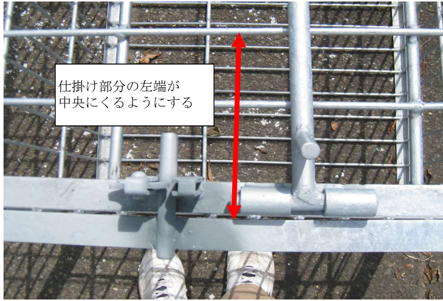
○上部からみた図面
