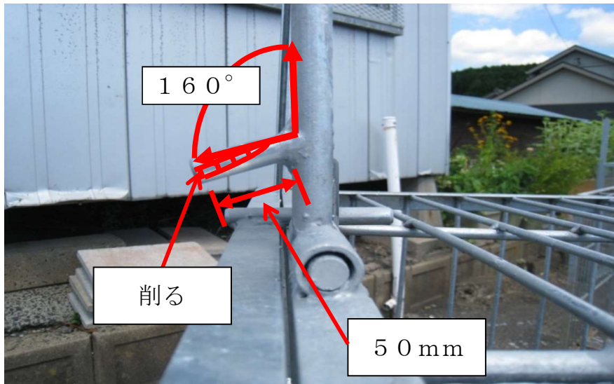
○側部からみた図面
