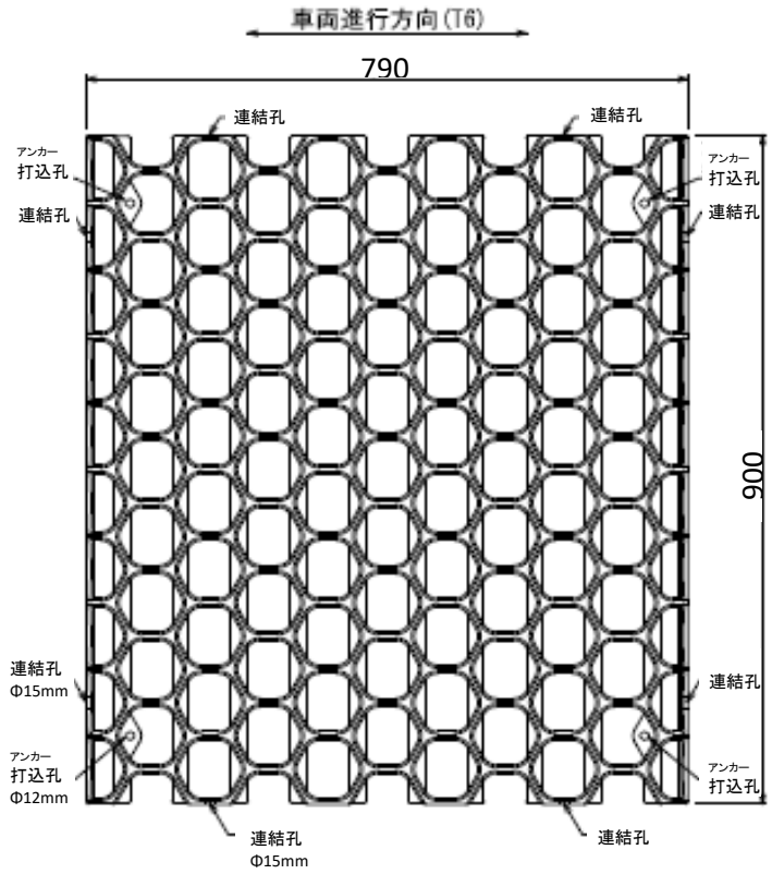
平面図
